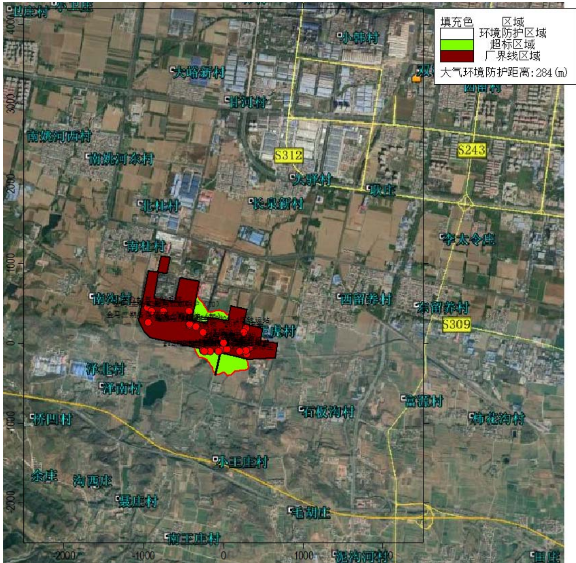
图 7.1-16 (2) (PM 10 ) 大气环境保护距离示意图
