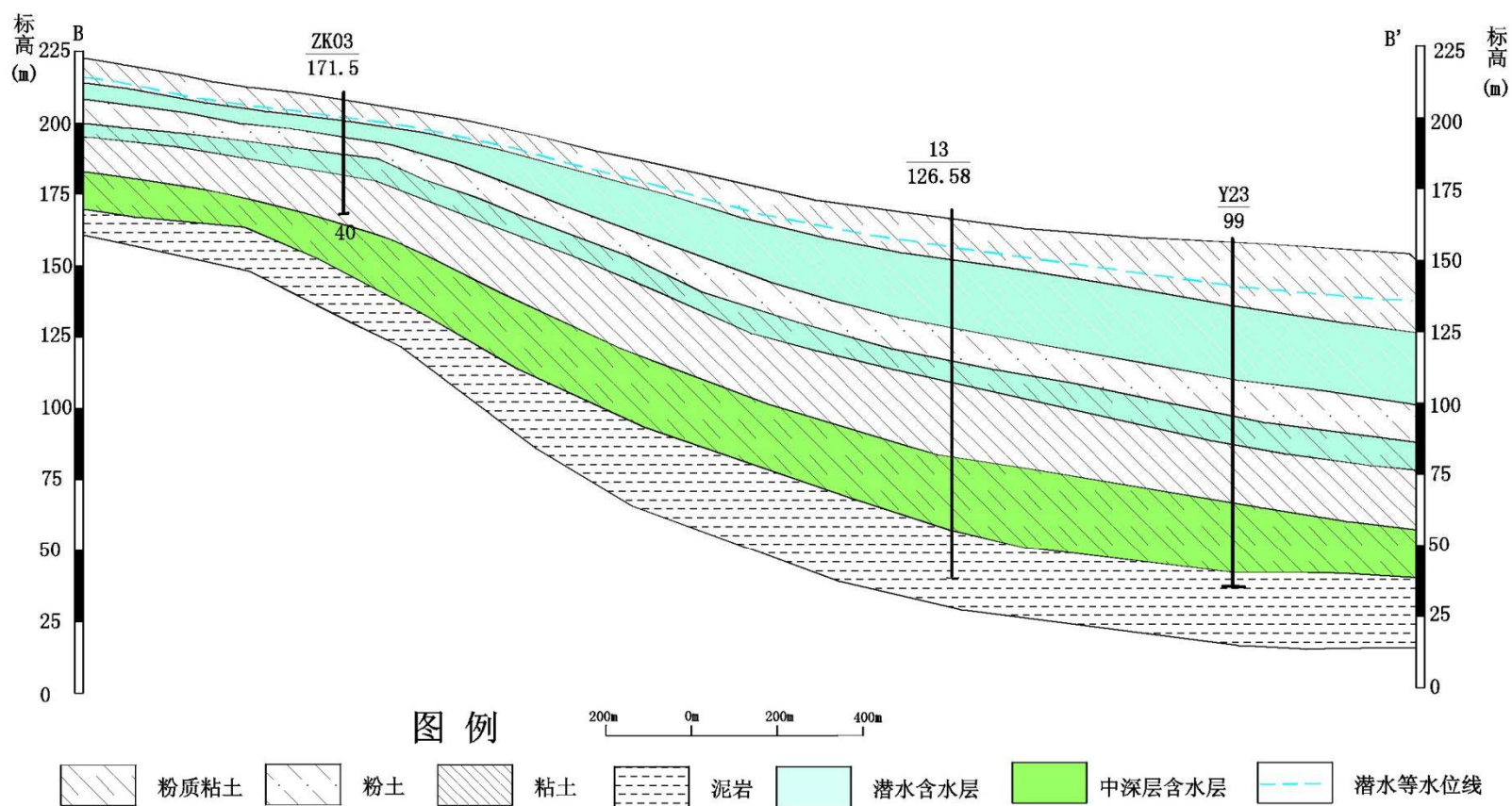
图 8.4-3 调查评价区 B-B' 水文地质剖面图
