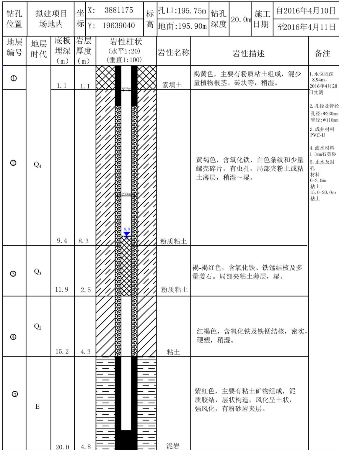
图 8.4-6 ZK01 钻孔柱状图
