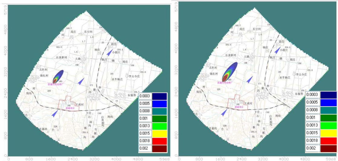
(1) 100 d 污染晕运移分布图
