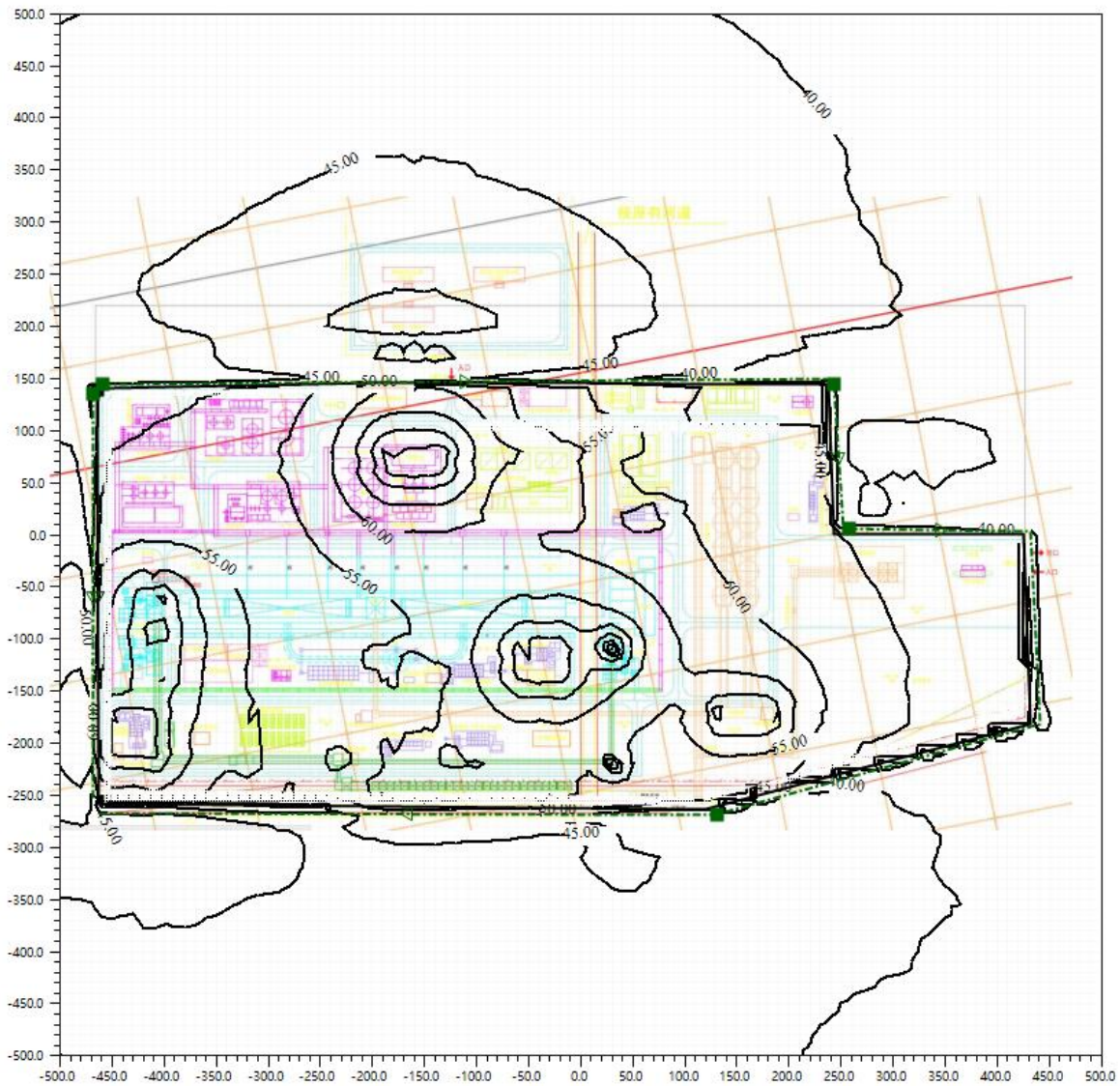
图 7.3-1 噪声贡献值等声级线图 (单位: dB (A))
