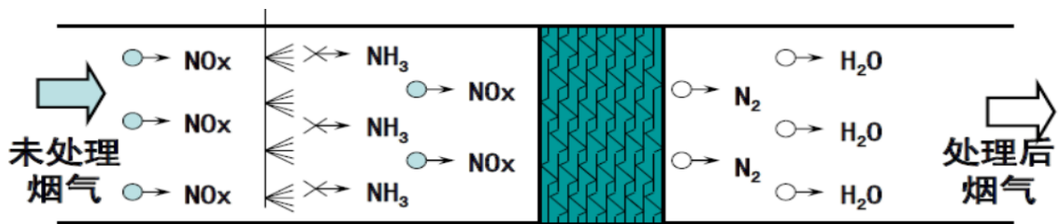
图 3.1-4 SCR 脱硝反应示意图
