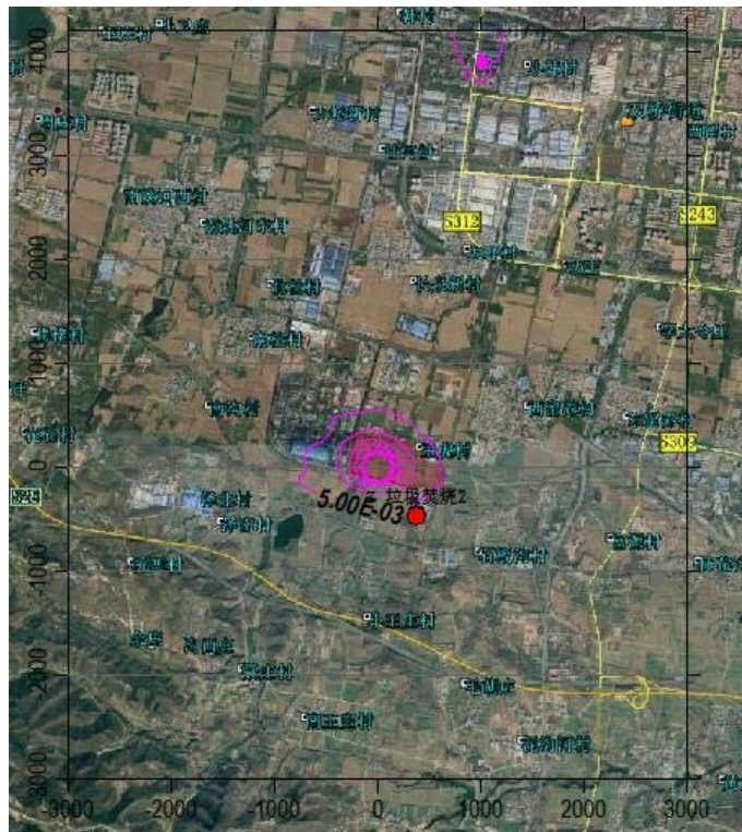
图 7.1-7 预测范围内 SO 2 第 98 百分位日均浓度叠加值分布图
