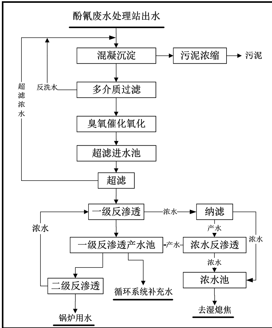
图 3.1-7 废水深度处理系统工艺流程
