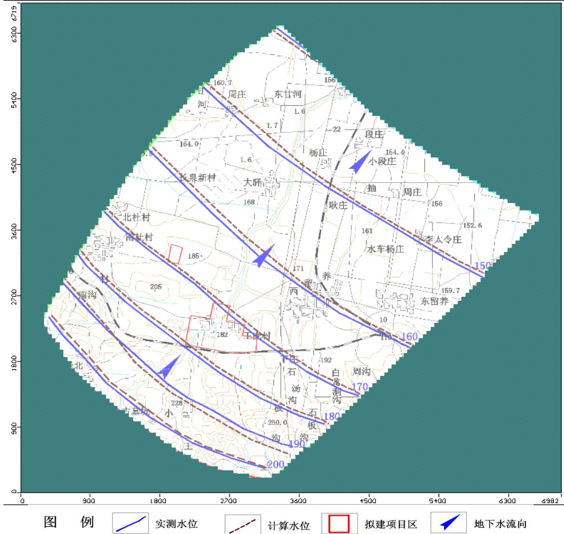
图 8.5-4 模型识别期流场拟合图
