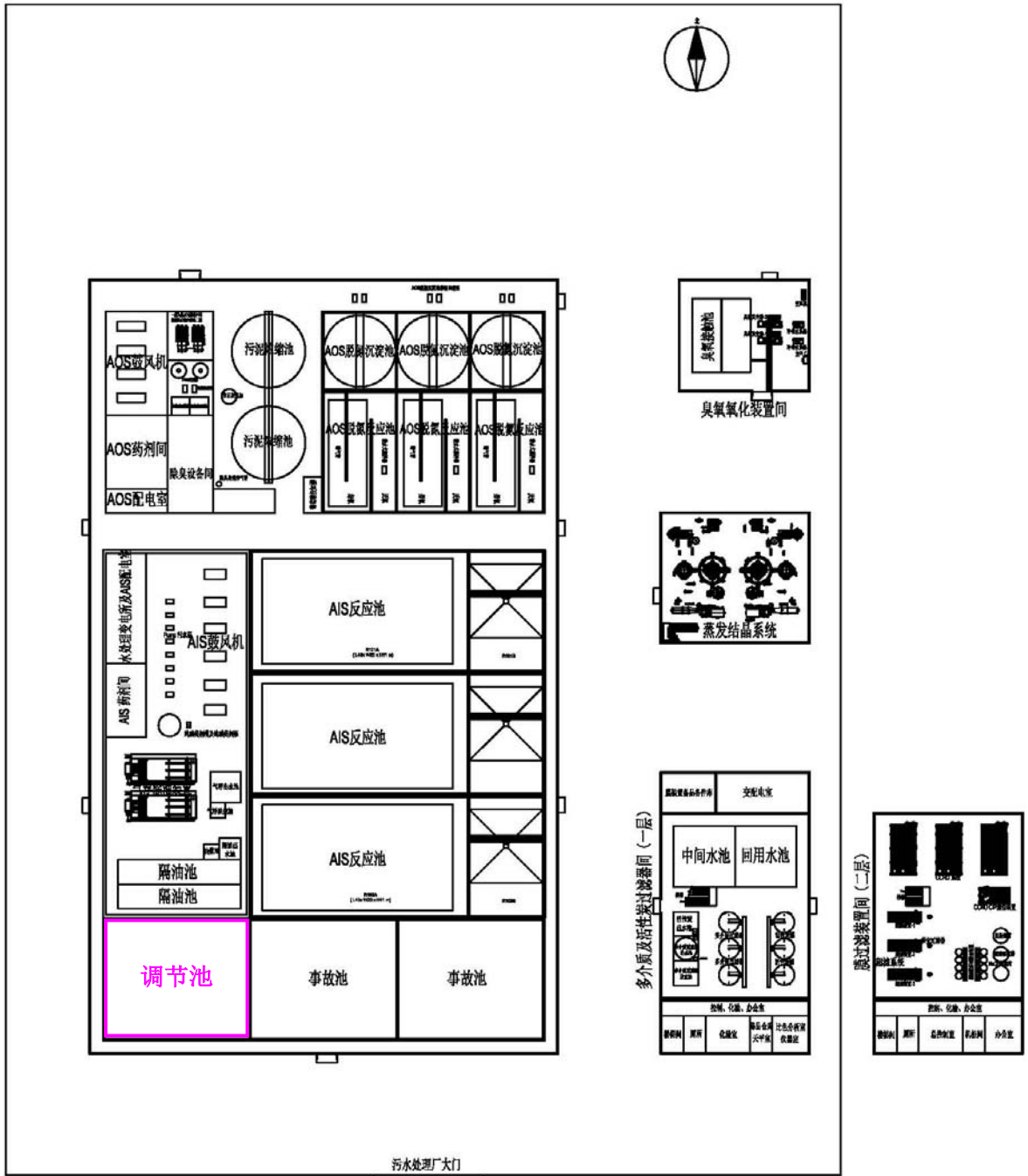
图9.6-2 (2) 厂区（酚氰废水处理站）危险单元分布示意图
