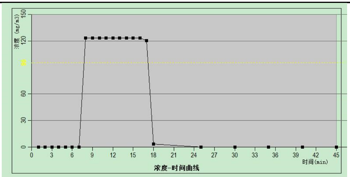
图 9.8-2 CO 浓度-时间变化情况示意图（小王庄）
