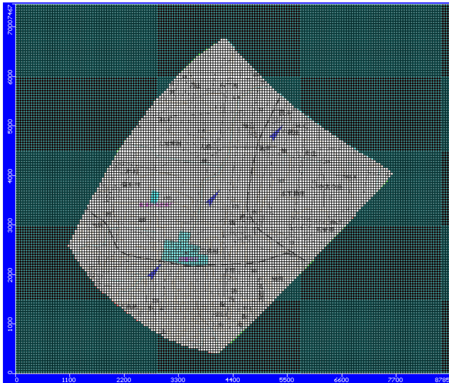
图 8.5-2 研究区网格剖分图
