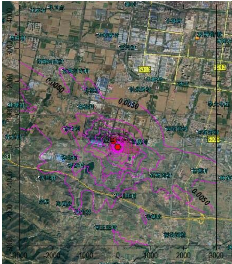
图 7.1-14 预测范围内苯小时浓度叠加值分布图 \text{mg}/\text{m}^3
