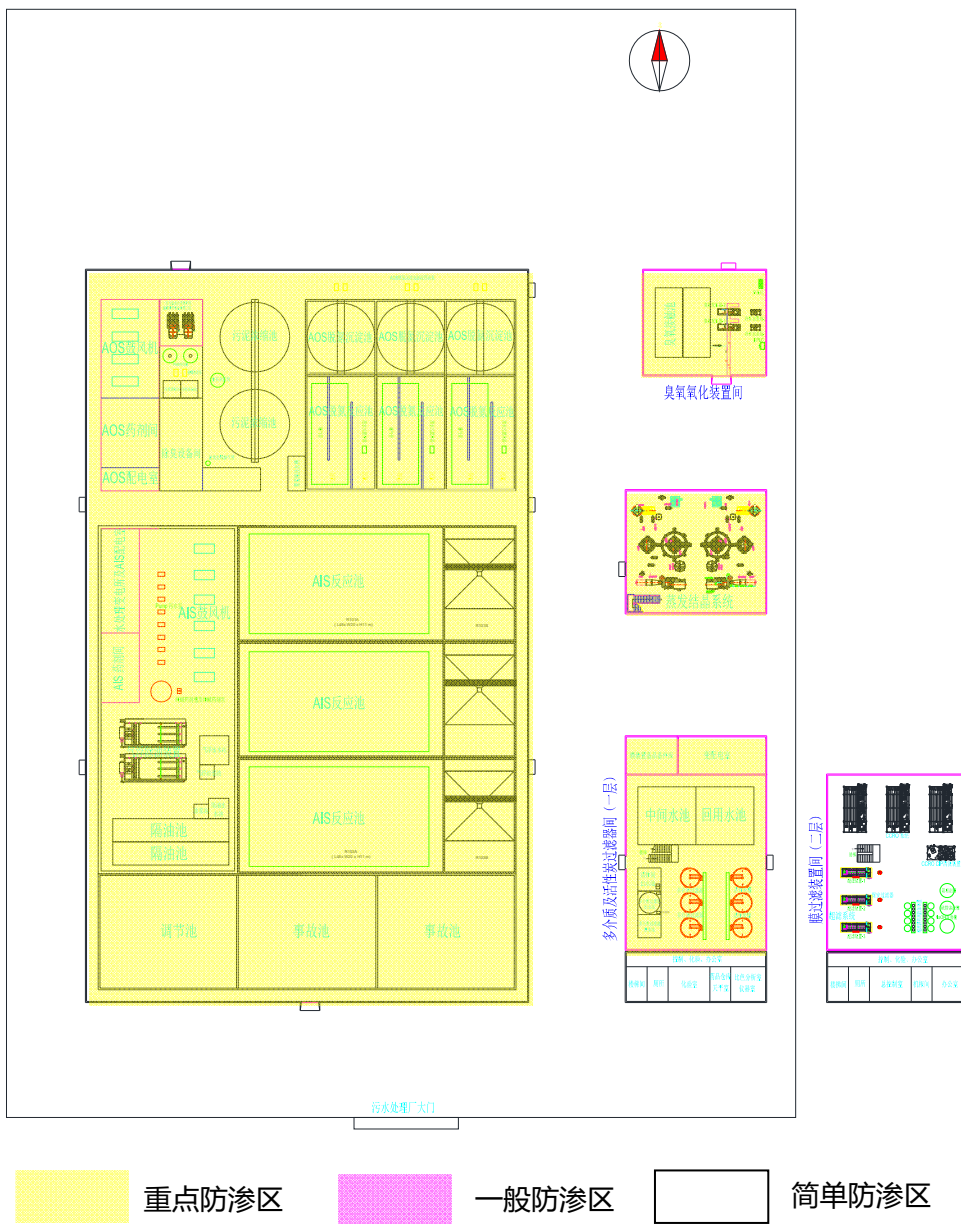
图 8.6-2 酚氰废水处理站分区防渗图
