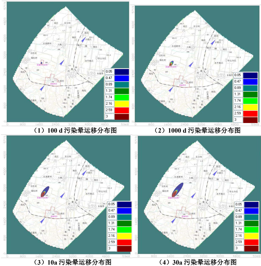
图 8.5-6 污染晕迁移分布图 (COD)
