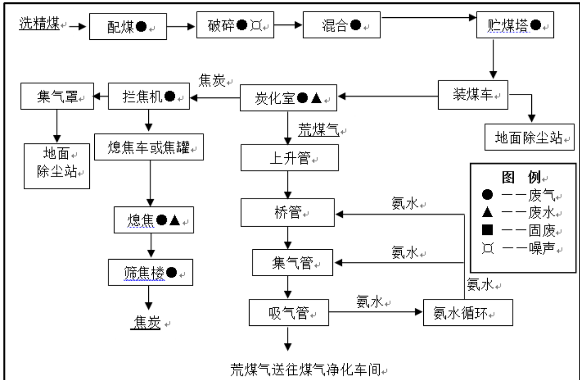
图 3.1-1 焦化工程工艺及产污节点图
