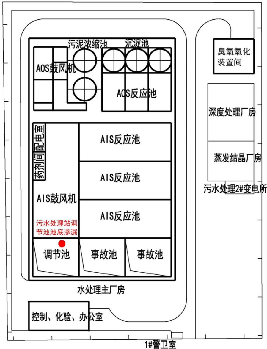
图 8.5-5 地下水污染预测泄漏点设定位置图
