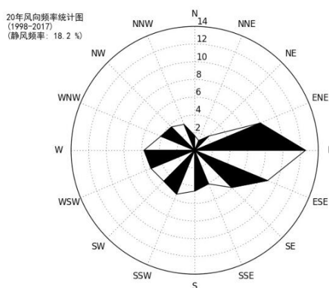
图 7.1-1 风频玫瑰图
